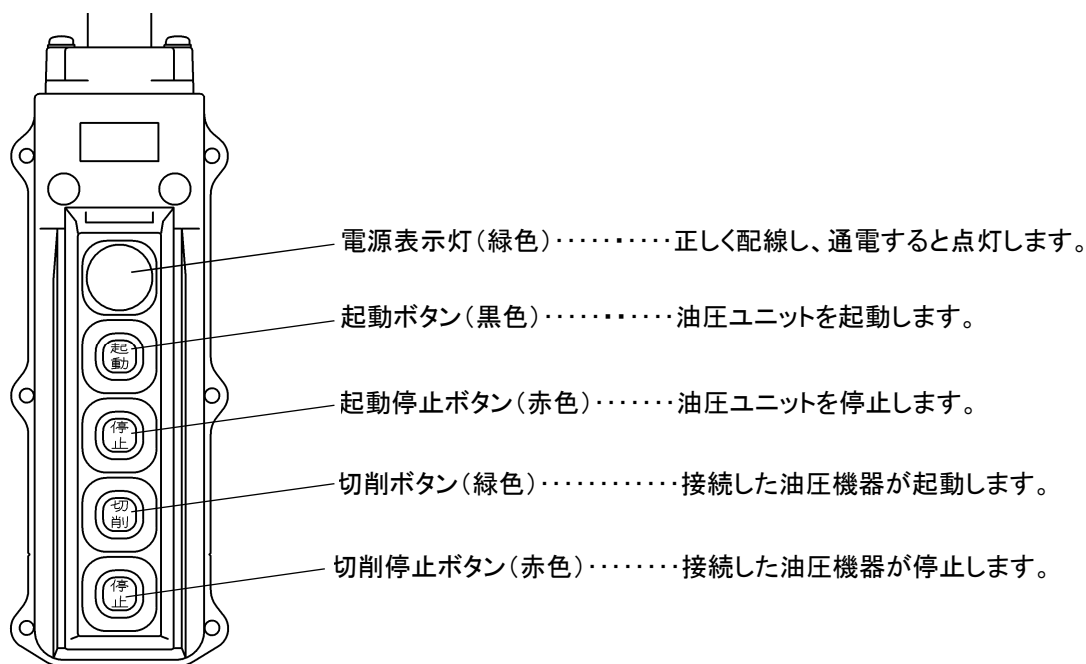
リモートコントロールスイッチ詳細 (ケーブル長20m)
